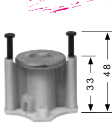
赤黄青緑 3分ボルト用(W3/8) 埋設深さ(30mm) 引抜強度: 17.70kN (1,800kgf)
