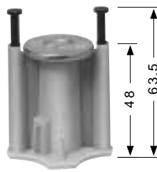
赤黄青 3分ボルト用(W3/8) (ロングタイプ) 埋設深さ(45mm) 引抜強度: 34.27kN (3,490kgf)
