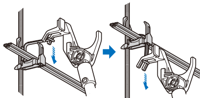
④結束バンドを締め付けます。(解除もできます。)
