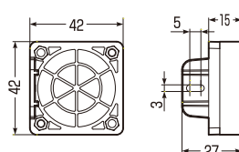
■換気扇本体
