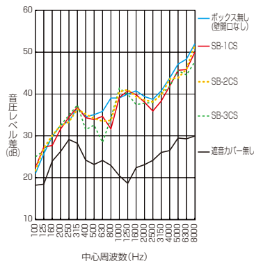
音圧レベル差試験
