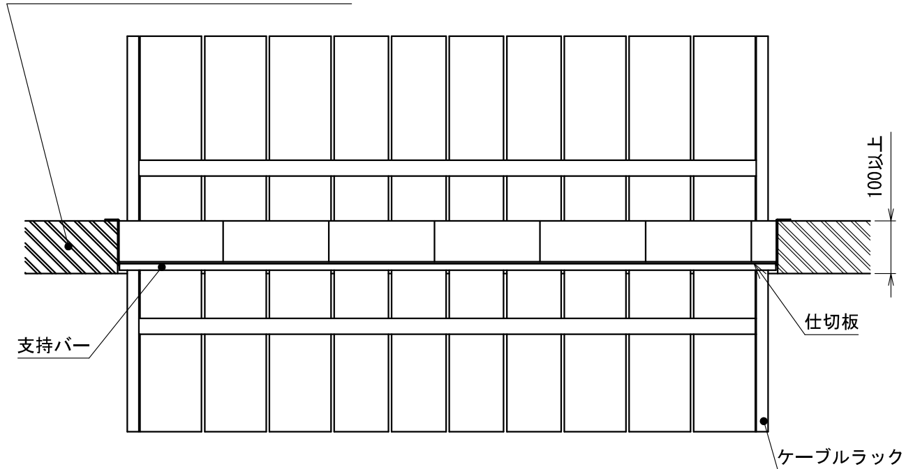
断面図
