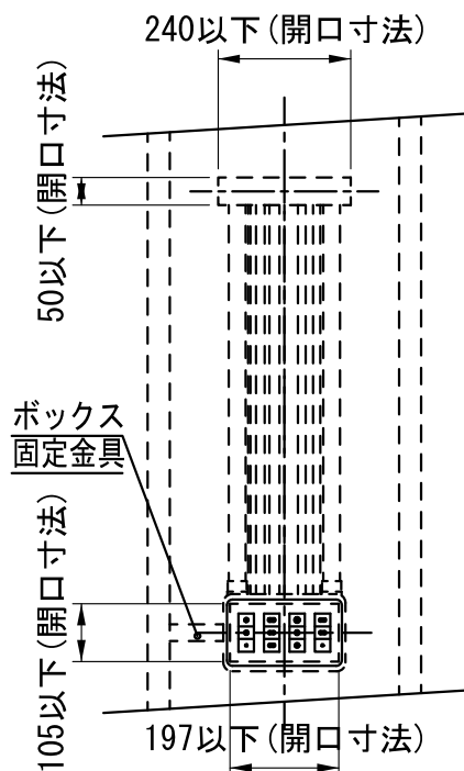
立面図(1/15) (ボックス固定金具を用いる場合)
