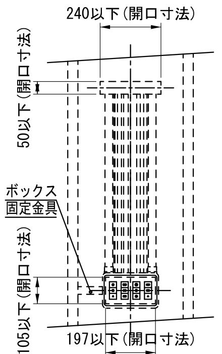
立面図(1/15) (ボックス固定金具を用いる場合)
