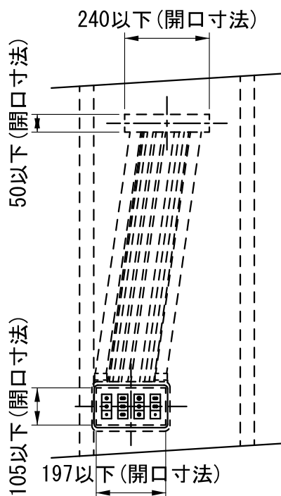
立面図(1/15) (ボックスを間柱に直付けする場合)
