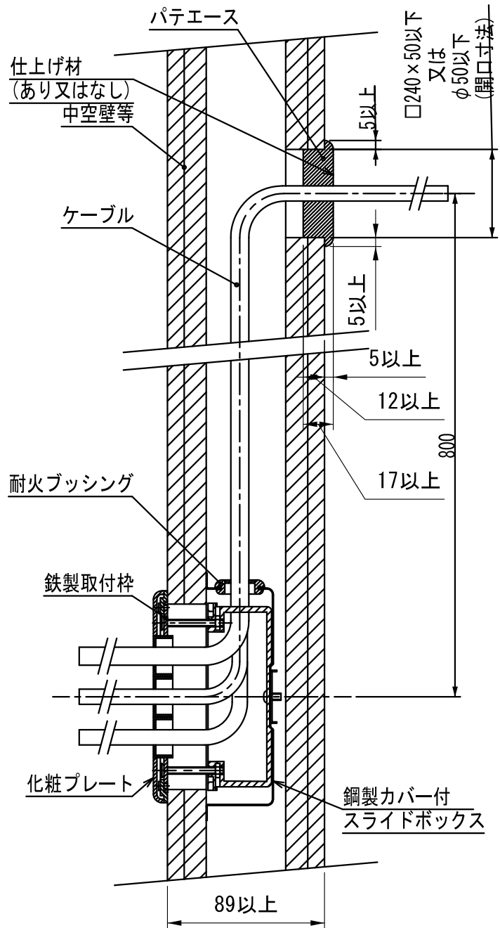
断面図 (1/3)
