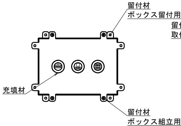
立面図(ボックス側)
