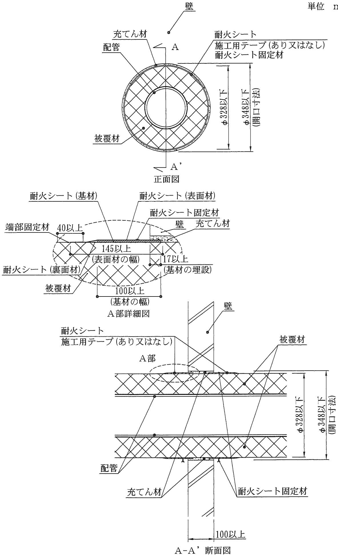
図1 構造説明図(施工図)
