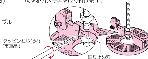
回り止め穴
